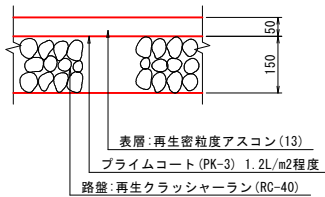
1号路肩舗装
