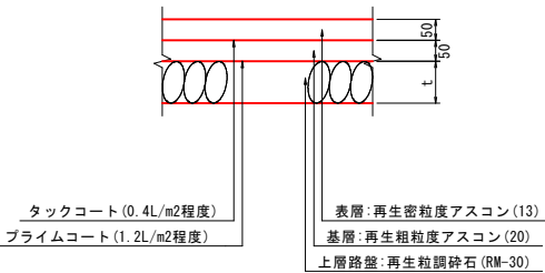
1号歩道舗装 (標準部)
