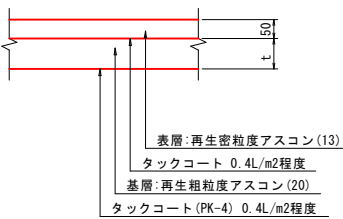
2号車道舗装
