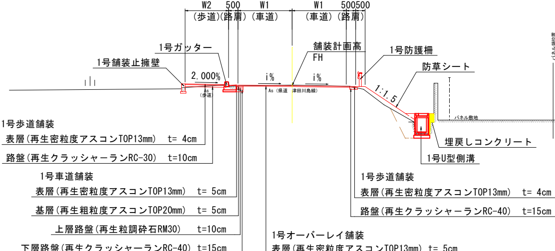
NO. 14付近 (一般部)
