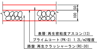
1号支道舗装
