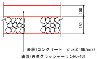
1号取合舗装
