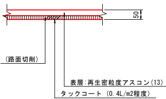
1号オーバーレイ舗装
