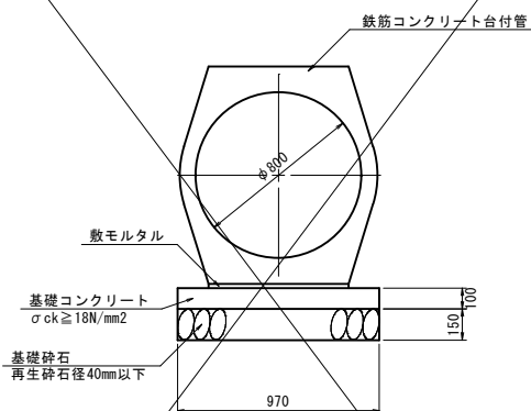
1号管渠 S=1:20 (鉄筋コンクリート台付管φ800)
