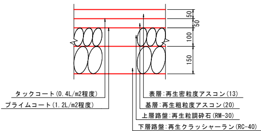
1号路肩舗装
