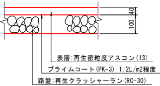
1号歩道舗装 (標準部)
